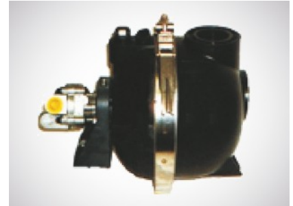
SW 1000 mit Hydraulikmotor
